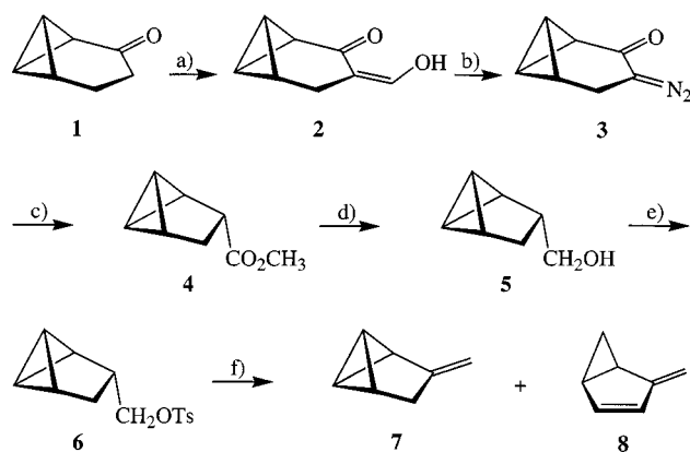
Scheme 1. a) \text{HCO}_2\text{Et} , \text{NaH}/\text{MeOH} , \text{Et}_2\text{O} , 20 °C; b) \text{TsN}_3 , \text{HNEt}_2 ; c) h\nu , \text{MeOH} ; d) \text{LiAlH}_4 , \text{Et}_2\text{O} ; e) \text{TsCl} , pyridine; f) \text{KOtBu} , \text{DMSO}
